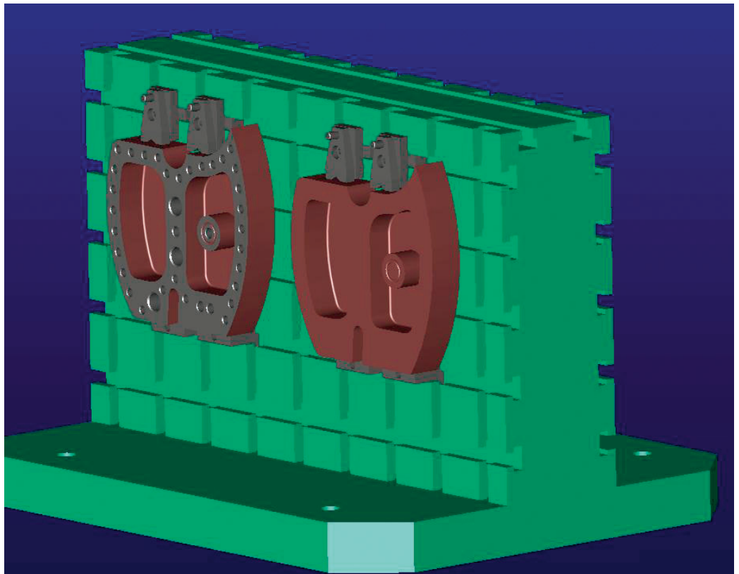
VALMIISTA KOMPONENTEISTA KASATTU PALETTI WINCAMILLA TYÖSTETTYINE KAPPALEINEEN.
