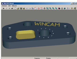
WINCAMILLA VISUALISOITU KAPPALE.
